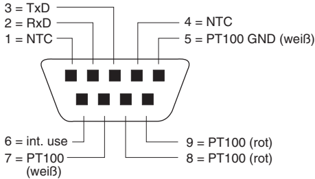
Pinbelegung RS232, DB9 Stecker
