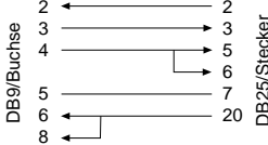
Com-Server -> Drucker W&T Art. Nr. 1189x
