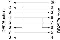
Com-Server <> PC, 25pol. W&T Art. Nr. 1179x
