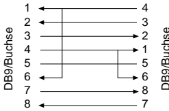
Com-Server <> PC, 9pol. W&T Art. Nr. 1199x
