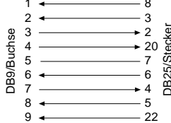
Com-Server <> Modem W&T Art. Nr. 1198x
