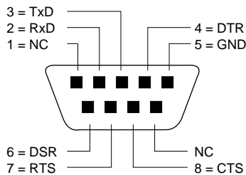
Pinbelegung RS232, DB9 Stecker
