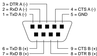
Pinbelegung RS422/485, DB9 Stecker
