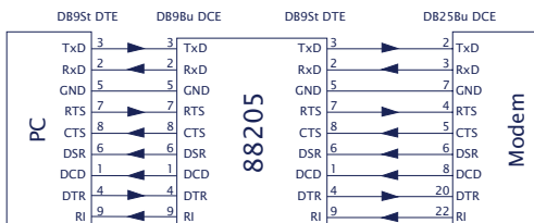
Galvanisch getrennte RS232-Verbindung mit Hardware-Handshake
