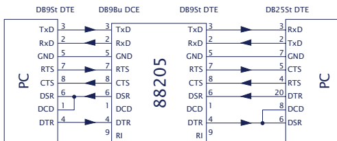
Galvanisch getrennte RS232-PC/PC-Kopplung mit Hardware-Handshake
