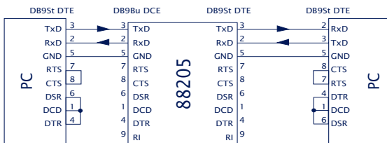
Galvanisch getrennte RS232-PC/PC-Kopplung mit Software-Handshake
