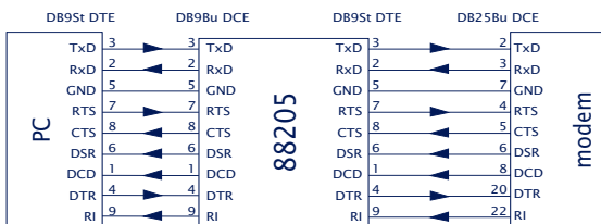
Galvanisch getrennte RS232-Verbindung mit Hardware-Handshake
