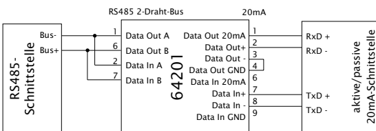
RS485 <> 20mA, Sendeschleife aktiv, Empfangsschleife passiv
