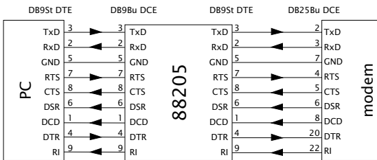
Galvanisch getrennte RS232-Verbindung mit Hardware-Handshake
