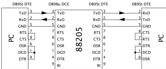
Galvanisch getrennte RS232-PC/PC-Kopplung mit Software-Handshake
