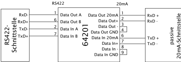
RS422 <> 20mA, Sende- und Empfangsschleife aktiv
