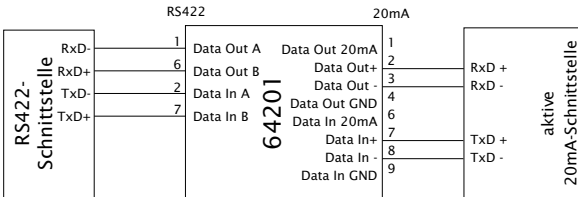
RS422 <> 20mA, Sende- und Empfangsschleife passiv
