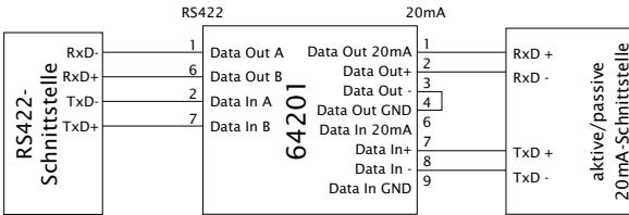
RS422 <> 20mA, Sendeschleife aktiv, Empfangsschleife passiv
