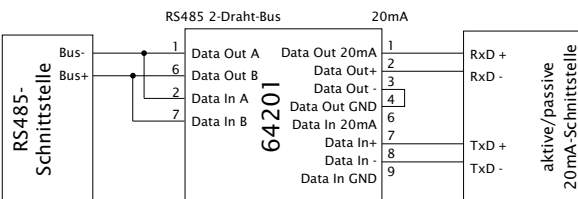
RS485 <> 20mA, Sendeschleife aktiv, Empfangsschleife passiv
