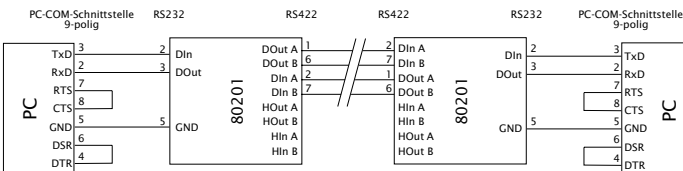
Bidirektionale RS232-Verbindung mit Software-Handshake
