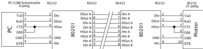
Bidirektionale RS232-Verbindung mit Hardware-Handshake
